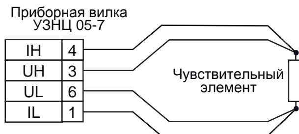
Рисунок Л.4 Электрическая схема ТСП-С
