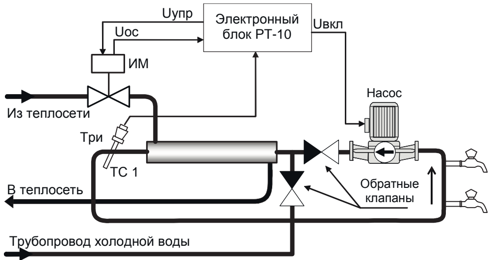
Рис.С.2 Узел приготовления теплоносителя системы ГВС с кожухотрубным теплообменником. Регулятор управляет двухходовым регулирующим клапаном по температуре Три (конфигурация 1) и циркуляционным насосом.
