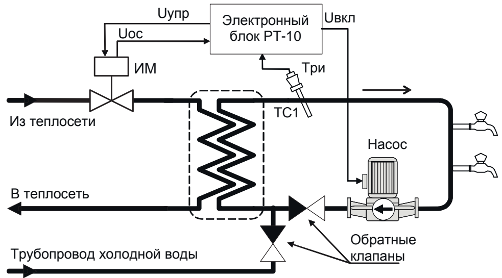
Рис.С.1 Узел приготовления теплоносителя системы ГВС с пластинчатым теплообменником. Регулятор управляет двухходовым регулирующим клапаном по температуре Три (конфигурация 1) и циркуляционным насосом.
